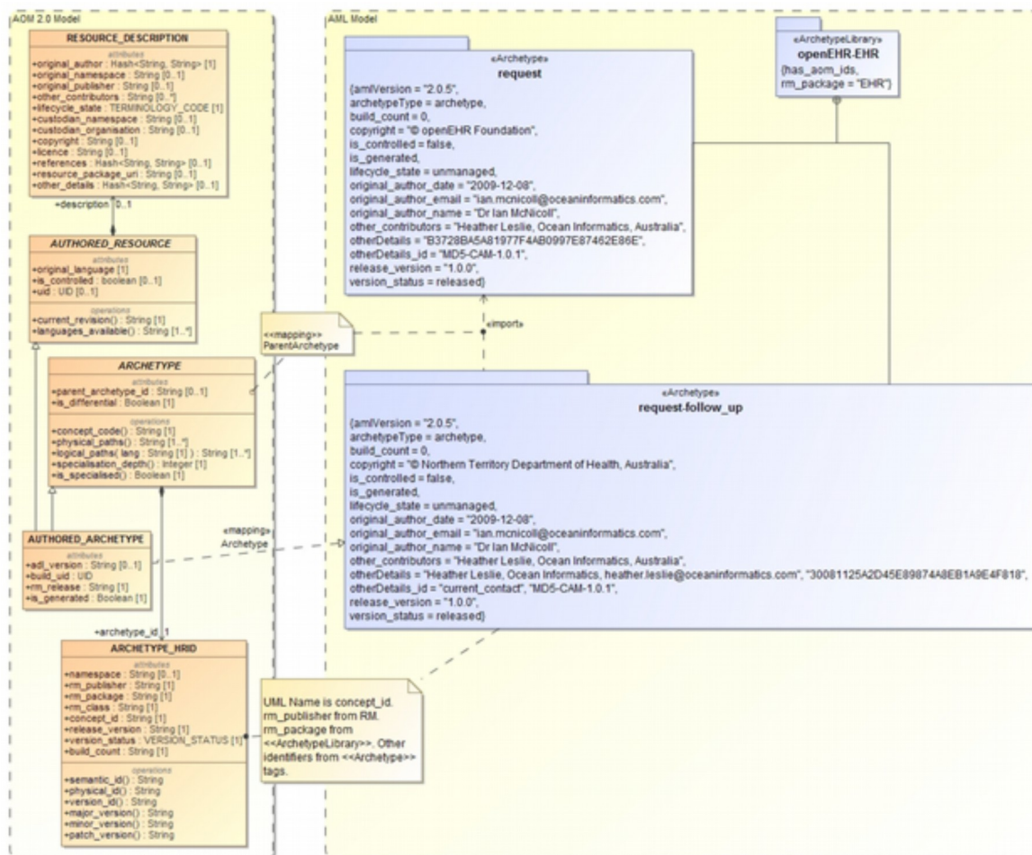
Figure 10. «Archetype» Mapping Overview
