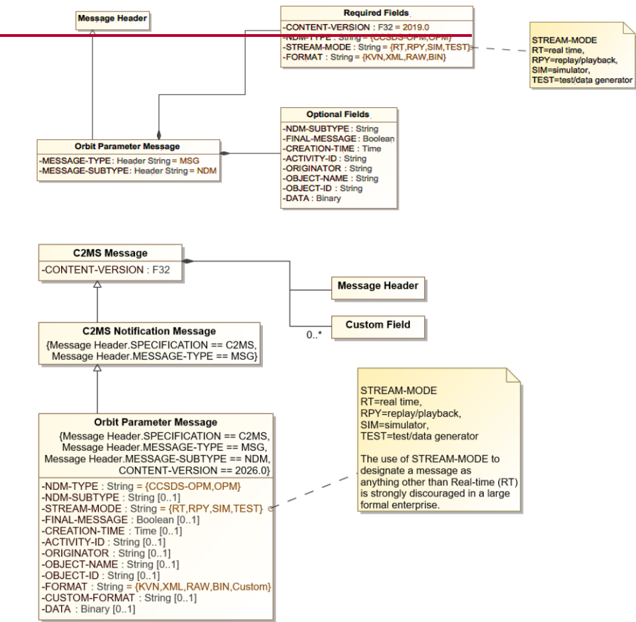
Figure 8-37. 8.45: Orbit Parameter Message Diagram
