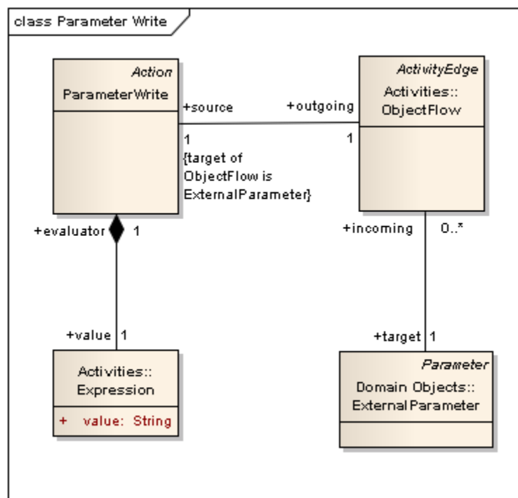
Figure 17: Parameter Write
