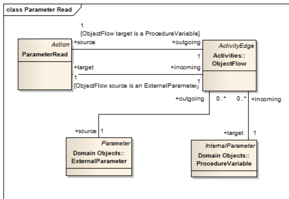
Figure 16: Parameter Read
