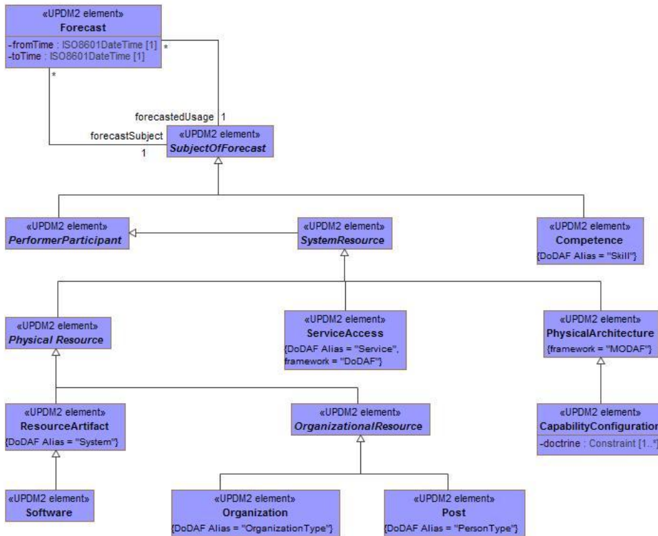
Figure A:44 - SV-9/SvcV-9 - DMM
