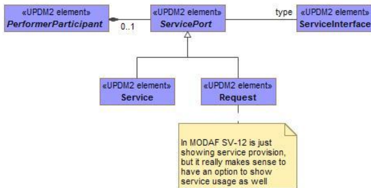
Figure A:36 - SV-12 - DMM
