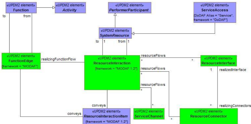
Figure A:41 - SV-6/SvcV-6 - DMM
