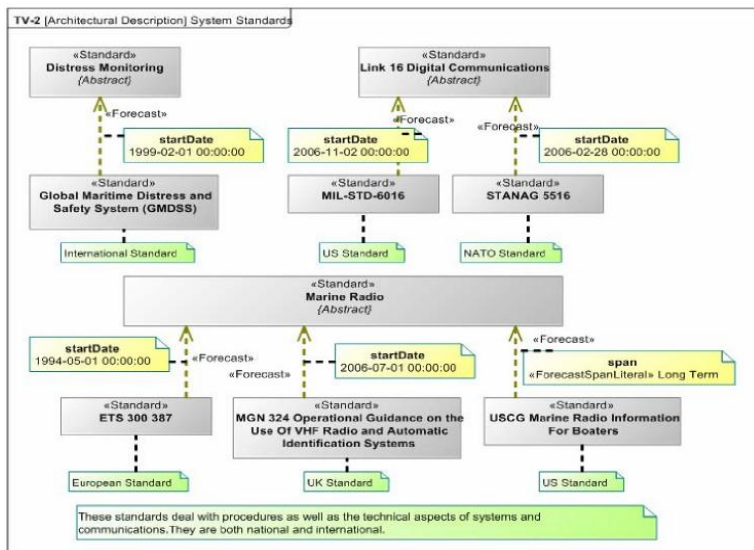
Figure D:45 - TV-2
