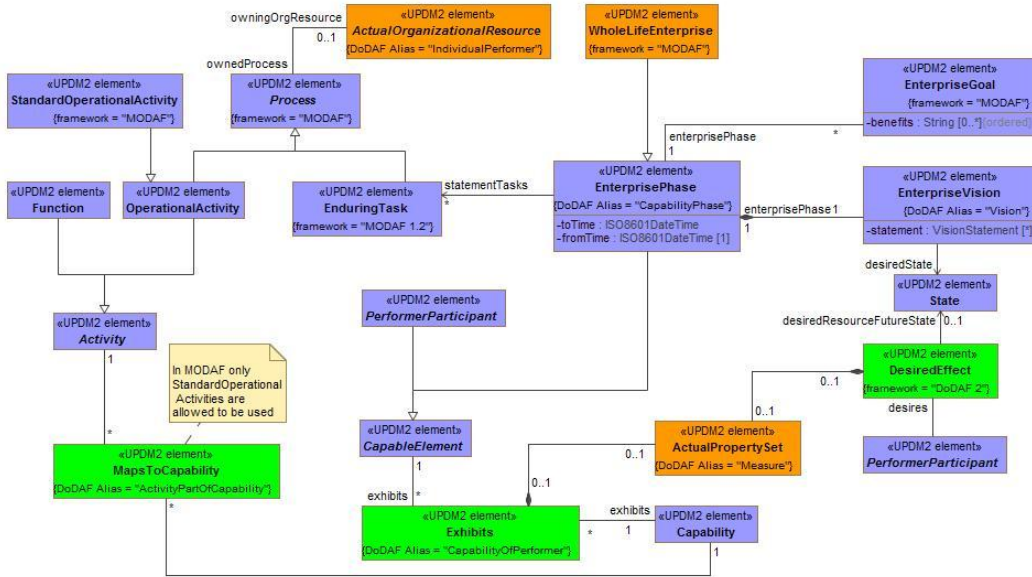
Figure A:25 - StV-1/CV-1 - DMM
