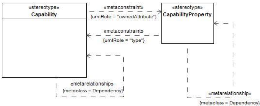
Figure B:30 - StV-4/CV-4
