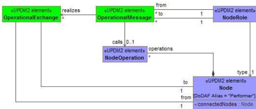
Figure A:15 - OV-6c - DMM
