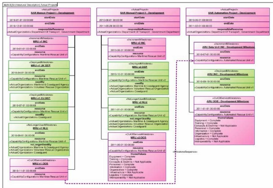
Figure D:42 - AcV-3 Actual
