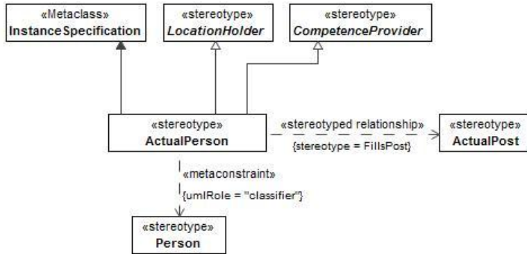
Figure 8:71 - ActualPerson
