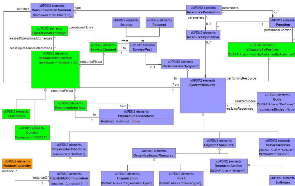
Figure A:31 - SV-1/SvcV-1 - DMM
