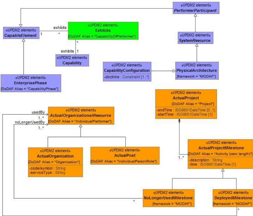
Figure A:29 - StV-5/CV-5 - DMM
