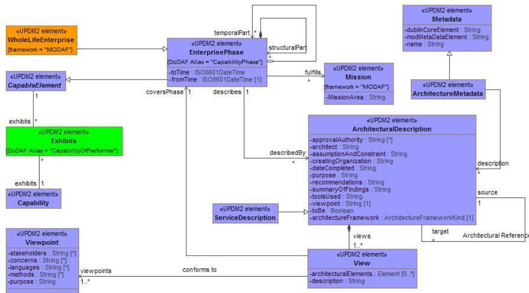
Figure A:5 - AV-1 - DMM
