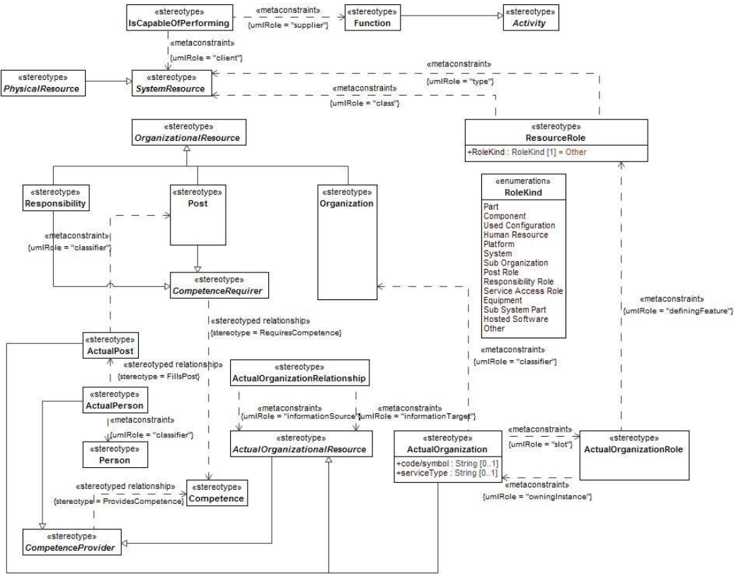
Figure B:12 - OV-4 Actual
