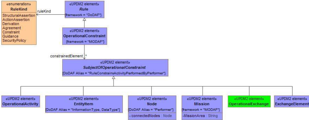
Figure A:13 - OV-6a - DMM
