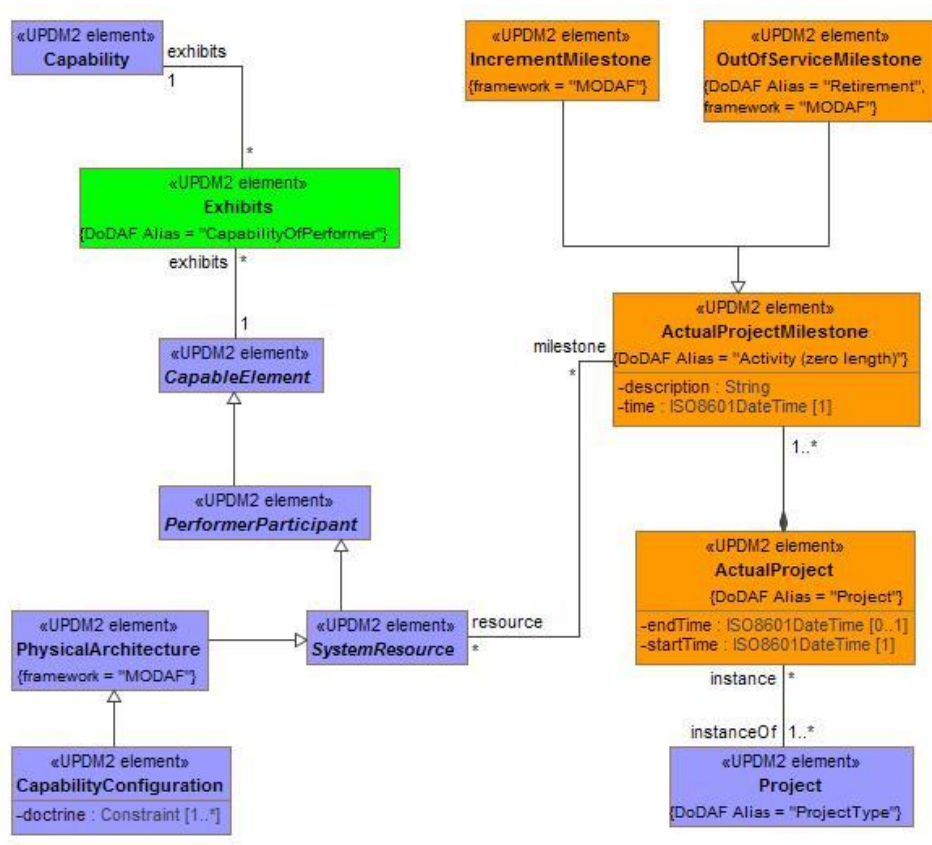
Figure A:27 - StV-3/CV-3 - DMM
