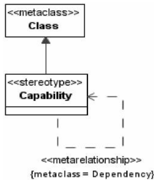
Figure 7:5 - Visualizing «metarelationship»
