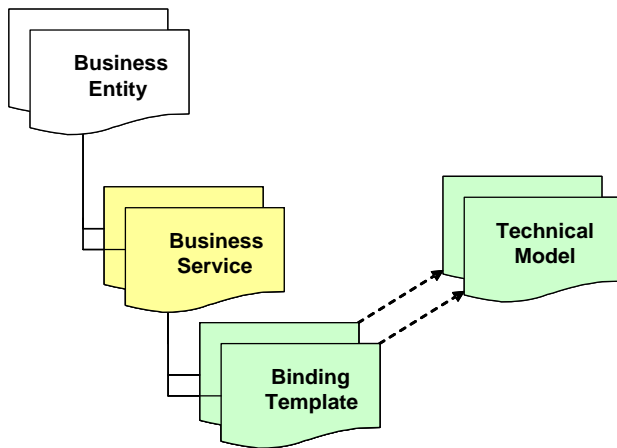
Figure 4: UDDI Overview
